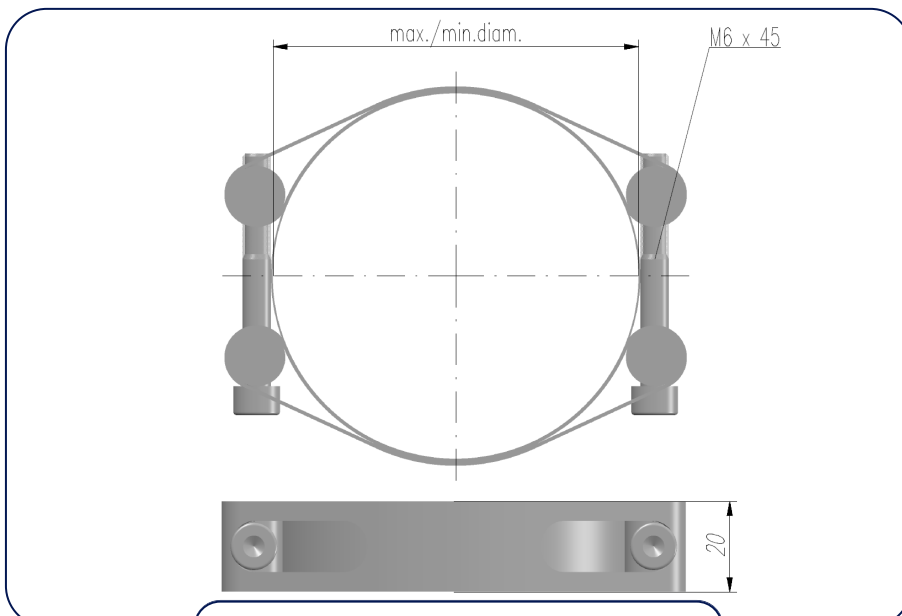
DIMENSIONS
