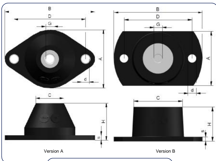
DIMENSIONS
