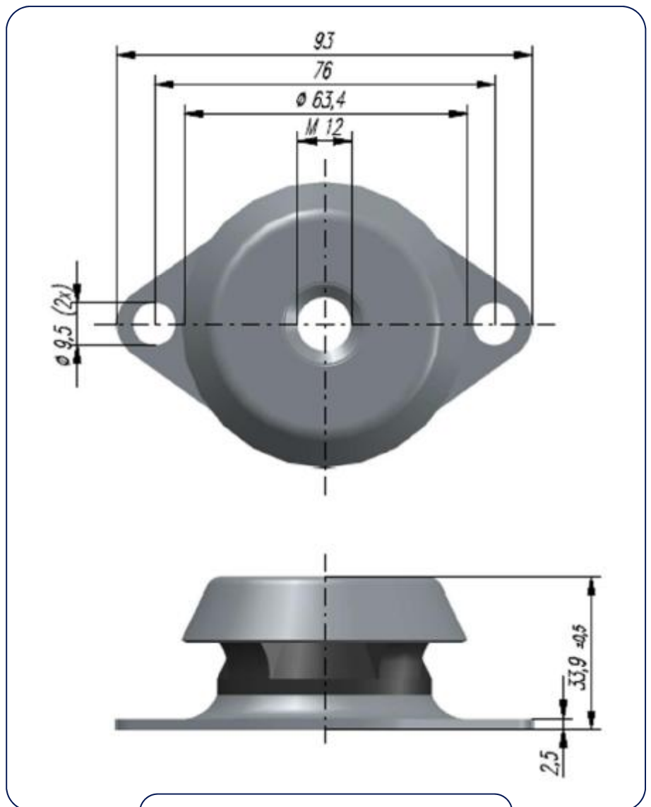
Dimensions
